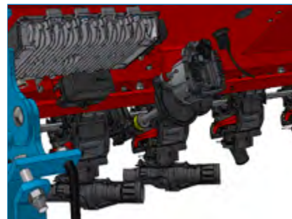
Fertiliseur FertiSmart Avec entraînement ISM (Integrated Smart Motors) Un moteur pour plusieurs doseurs
